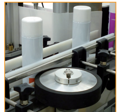
Spacer by motorized wheel Distanziatore a ruota motorizzata
